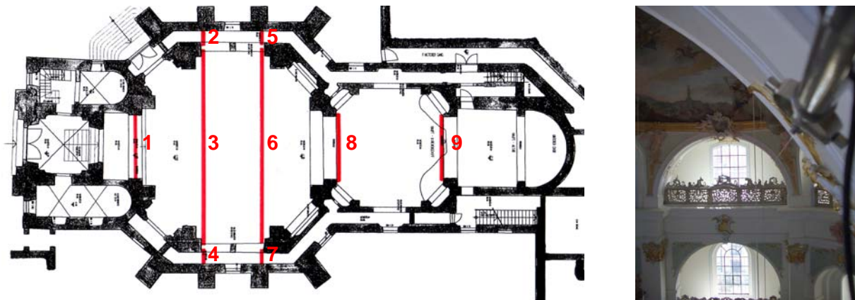
Abb. 3a & 3b: Digitales Konvergenzmesssystem mit Invardrähten in der Klosterkirche Altomünster
