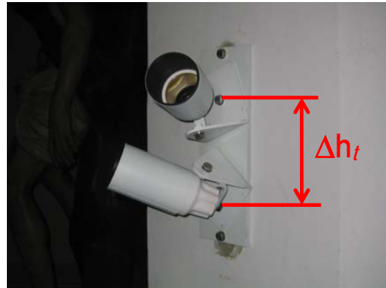
Abb. 10b) Kombiniertes Objekt-/Verknüpfungspunkt (Doppelprisma vertikal übereinander auf gemeinsamer Grundplatte, kann von mehreren Tachymetern gleichzeitig angezielt werden, \Delta h_t = 100 \text{ mm} = \text{const.} )
