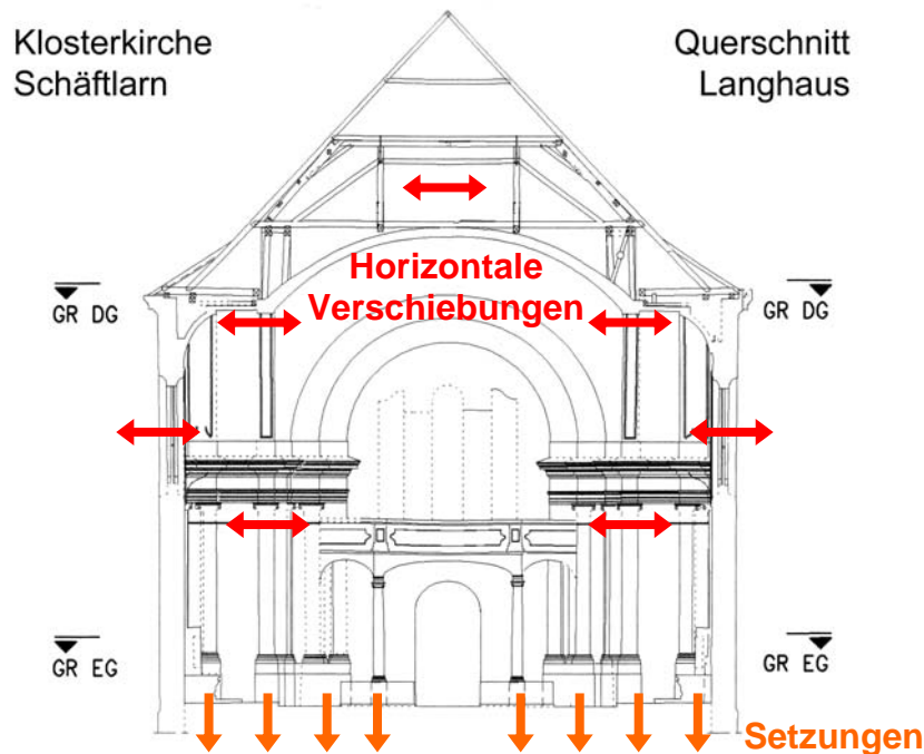
Abb. 1: Ungleichmäßige Setzungen historischer Bauwerke führen oft zu horizontalen Verschiebungen und somit zu Rissbildungen oder sogar größeren Schäden
