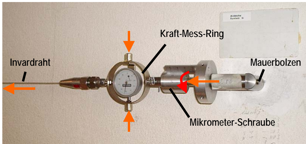
Abb. 2: Analoge Messuhr zum Konvergenzmesssystem mit Invardrähten
