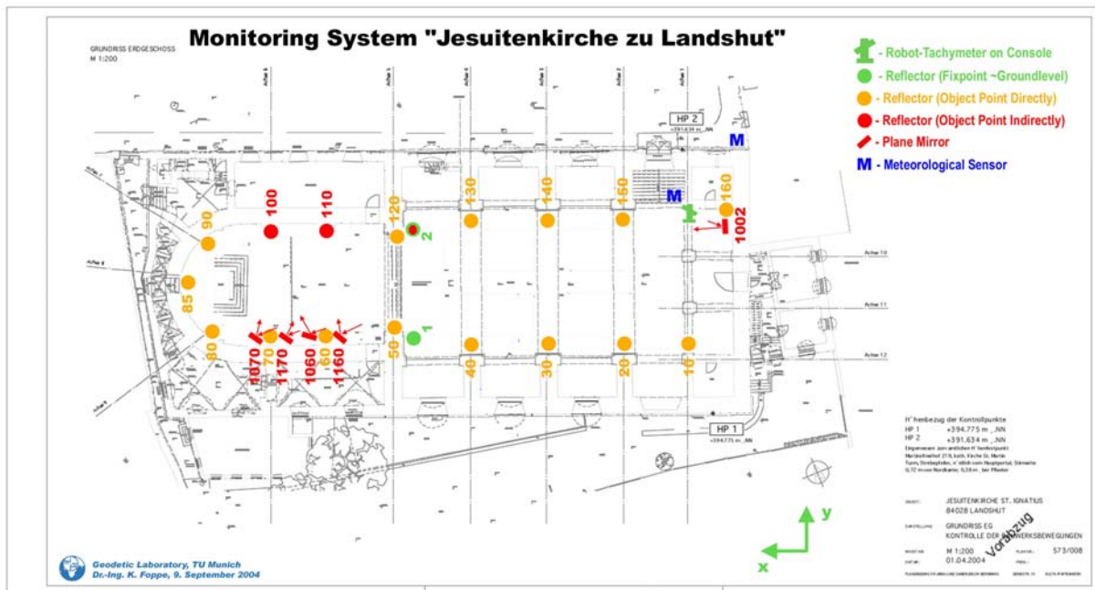
Abb. 11: Beispiel zum Aufbau eines Monitoring Systems in einem historischen Bauwerk ( Jesuitenkirche zu Lansdhut )
