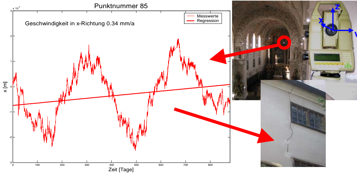
Abb. 16: Trends über zwei Jahren erklären die Rissbildung ( Jesuitenkirche zu Landshut )
