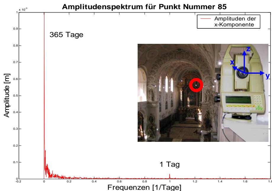
Abb. 17: Die Frequenzen 1 Tag und 365 Tage weisen auf die Temperatur als Haupteinflussgröße hin ( Jesuitenkirche zu Lansdhut )
